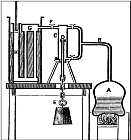
James Watt sukurtas aparatas.
